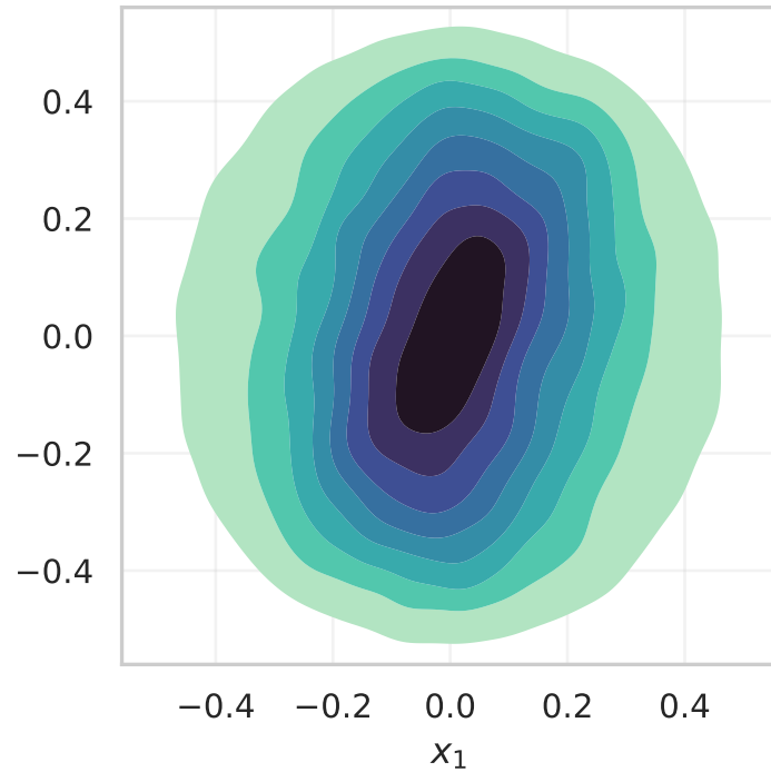
J_s, s=16
