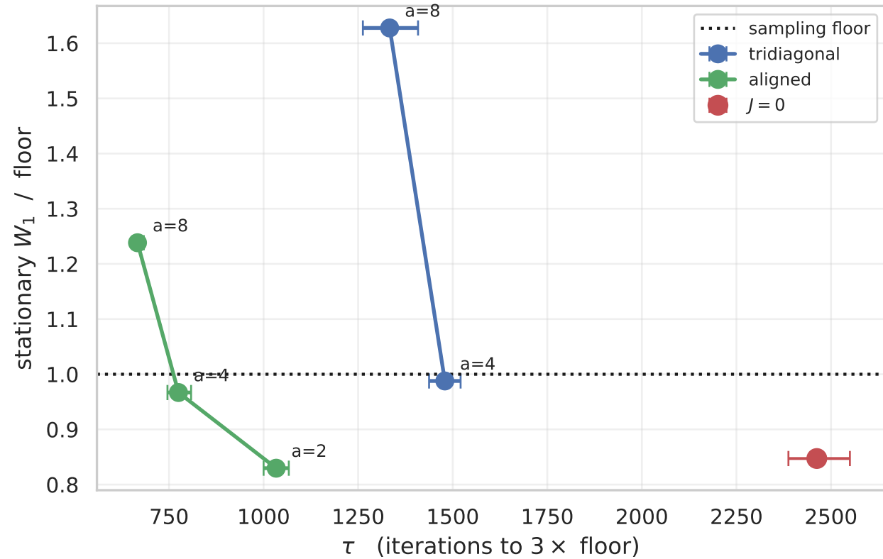
Target A: elliptical Laplace
