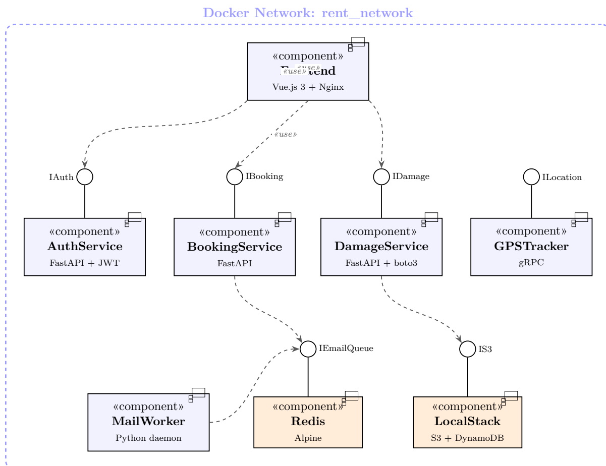
Slika 2: UML dijagram komponenti sustava RS-Rently
