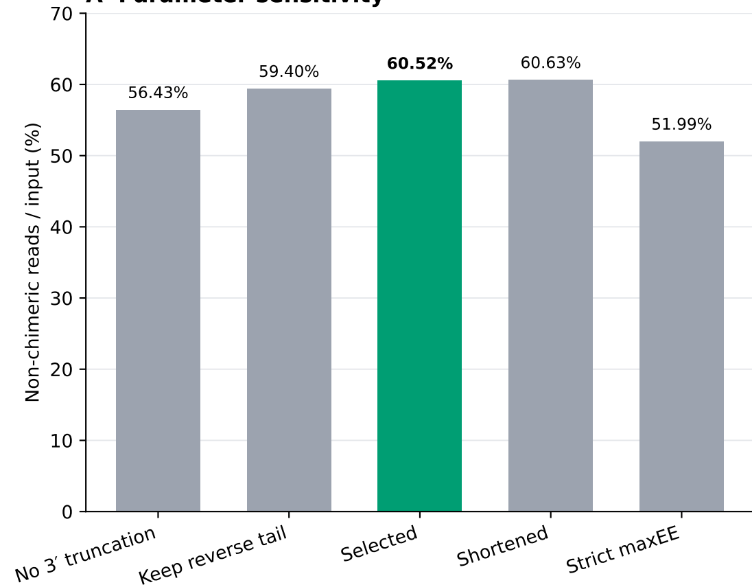
A Parameter sensitivity
