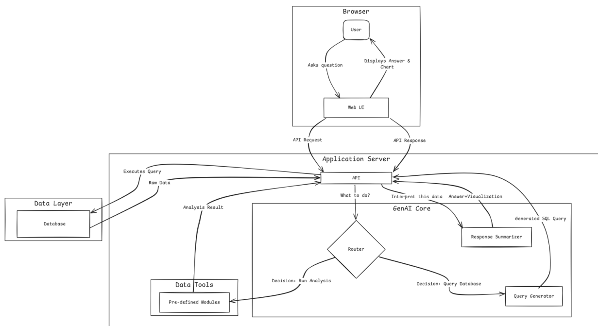
Obr. 1: Vysokoúrovňová architektúra systému
