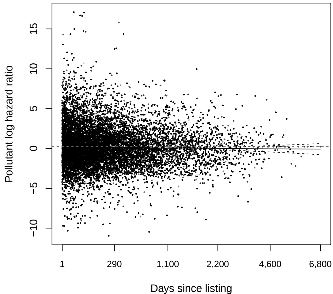
Heart PM 2.5
