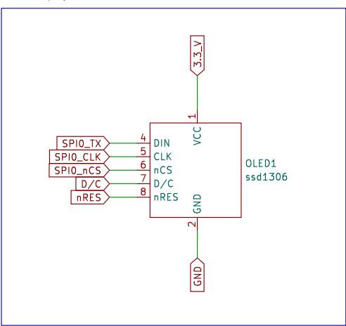
OLED display
