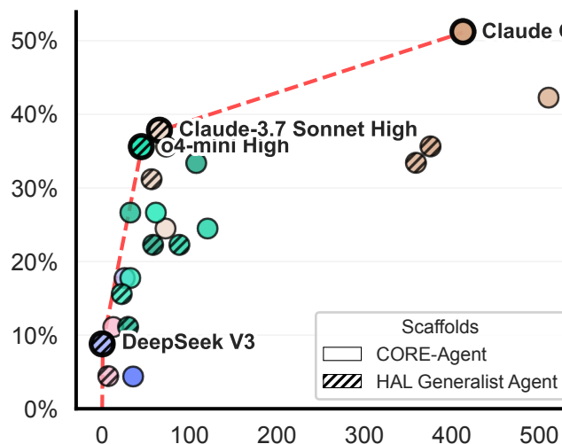
SWE-bench Verified Mini
