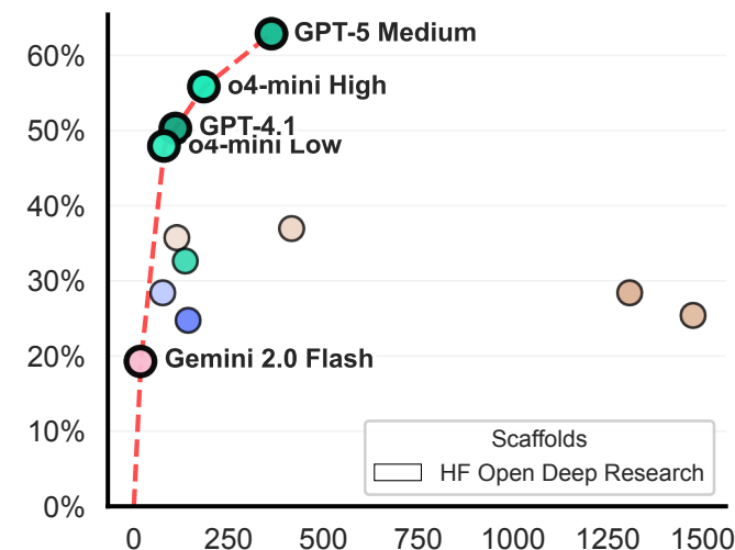
SciCode
