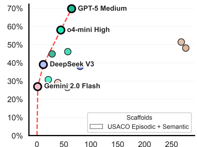
USACO
