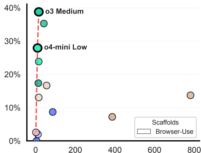
Online Mind2Web
