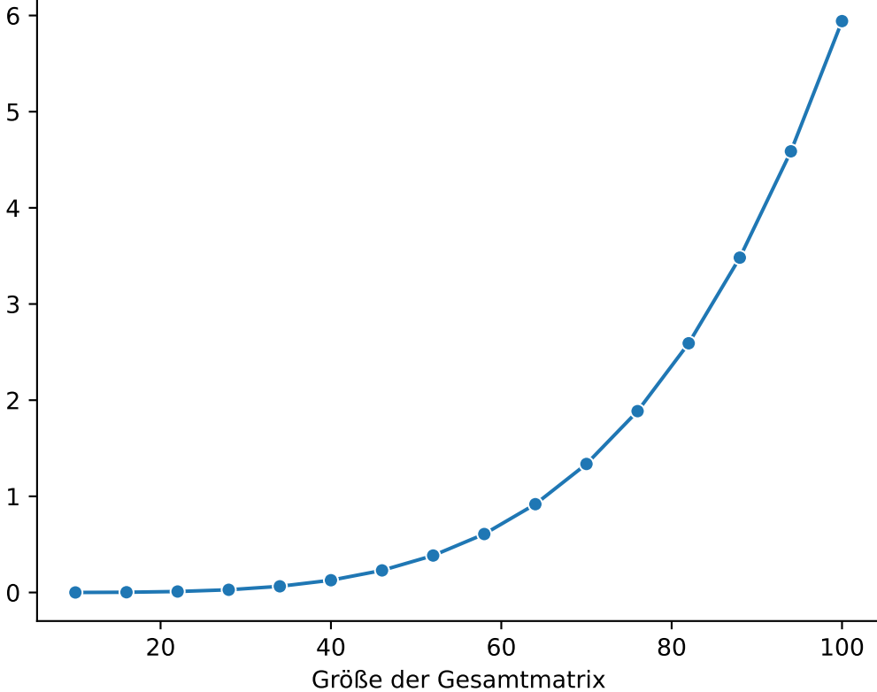
Annäherung an die Mischzeit bei Modell 2
