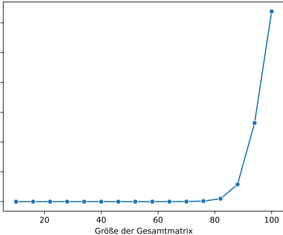
Annäherung an die Mischzeit bei Modell 3
