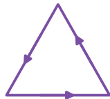
N_0 Nédélec
