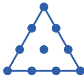
P_3 Lagrange
