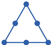
P_2 Lagrange
