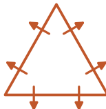
BDM_1
