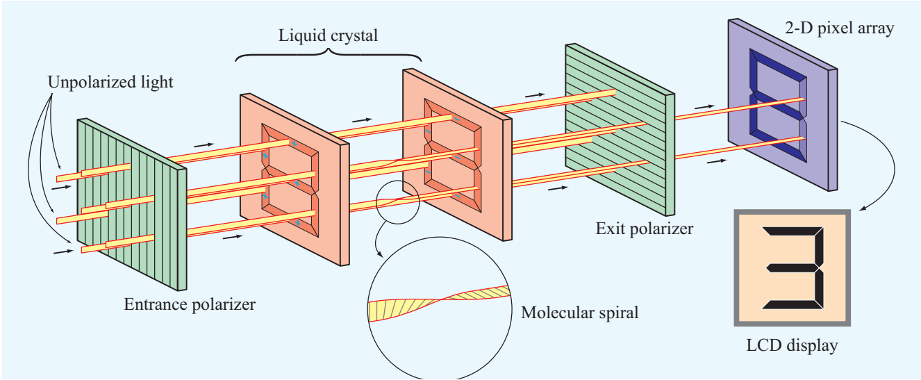
图 1-1 二维液晶显示阵列。
