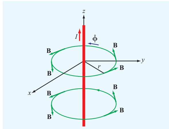
图1-9 沿 z 方向的恒定电流产生的磁场。
