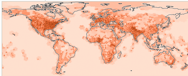
News events: posterior mean rate
