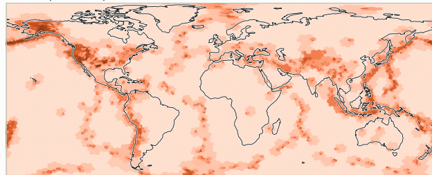
Earthquakes: posterior mean rate
