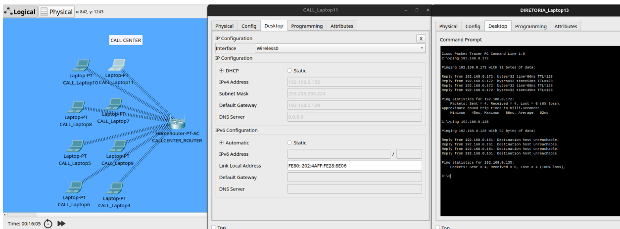
Figura 8: Laptops de diferentes rede Wireless em teste de ping.
