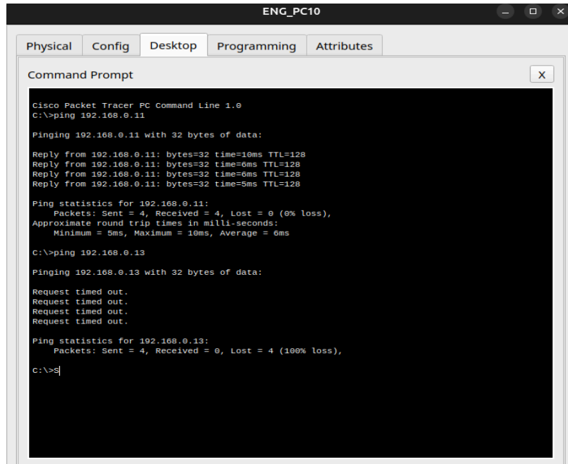
Figura 5: Teste de ping entre computadores de iguais e diferentes VLANs
