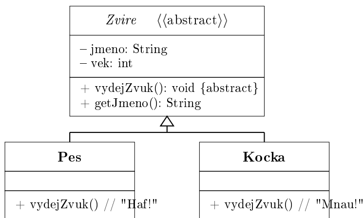
Obrázek 2: Ukázka diagramu tříd – hierarchie zvířat
