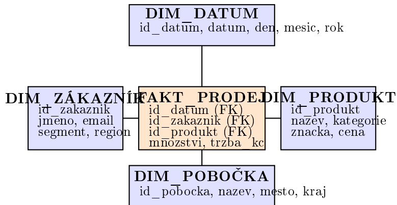
Obrázek 6: Hvězdicové schéma (Star Schema) – e-shop prodeje
