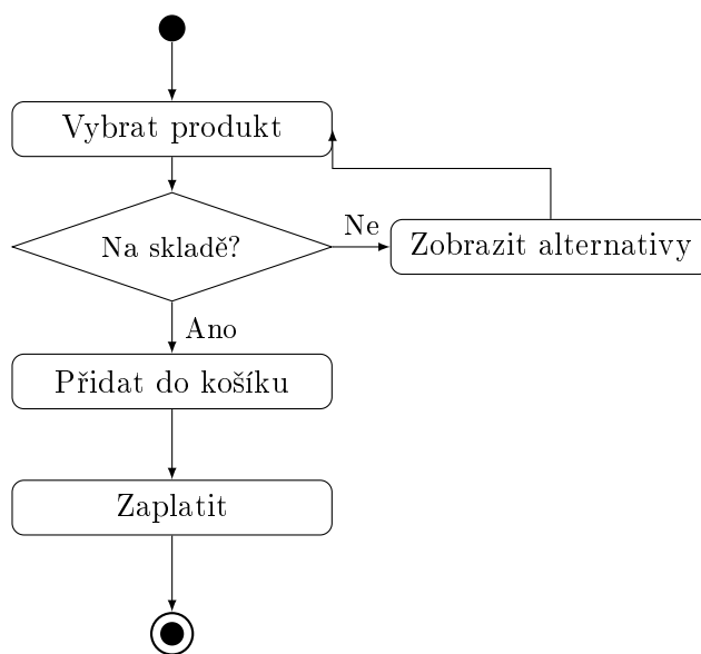
Obrázek 4: Ukázka diagramu aktivit – proces objednávky
