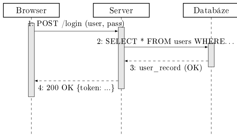
Obrázek 3: Ukázka sekvenčního diagramu – přihlášení uživatele
