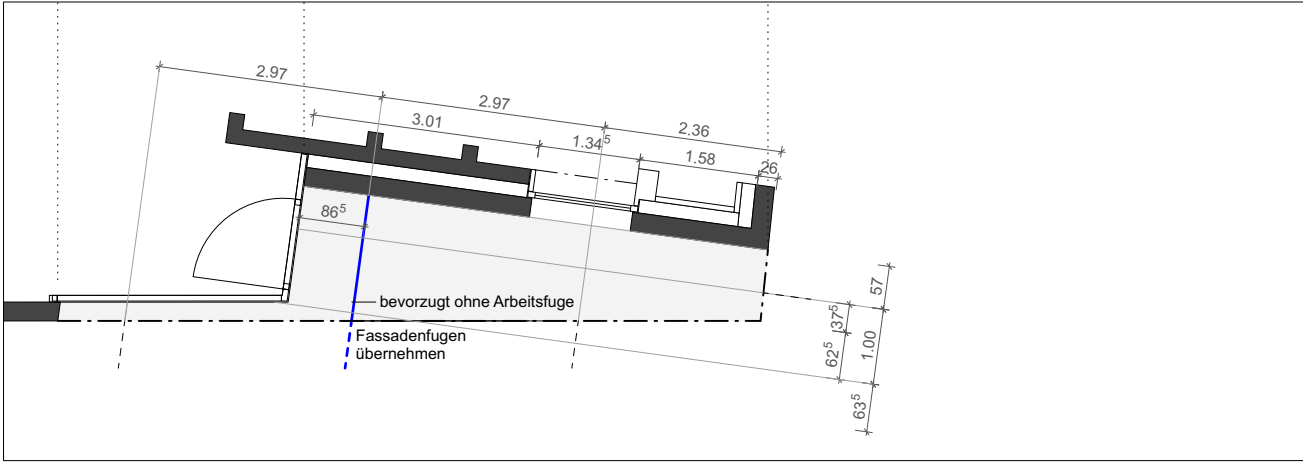
Deckenspiegel über EG
