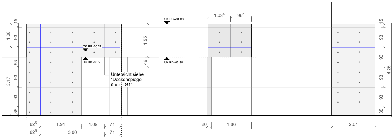
Ansicht Nord
