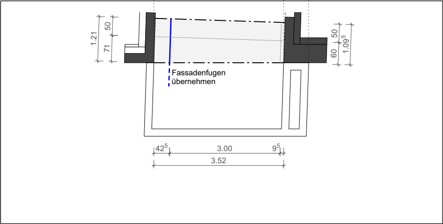
Deckenspiegel über Balkon EG
