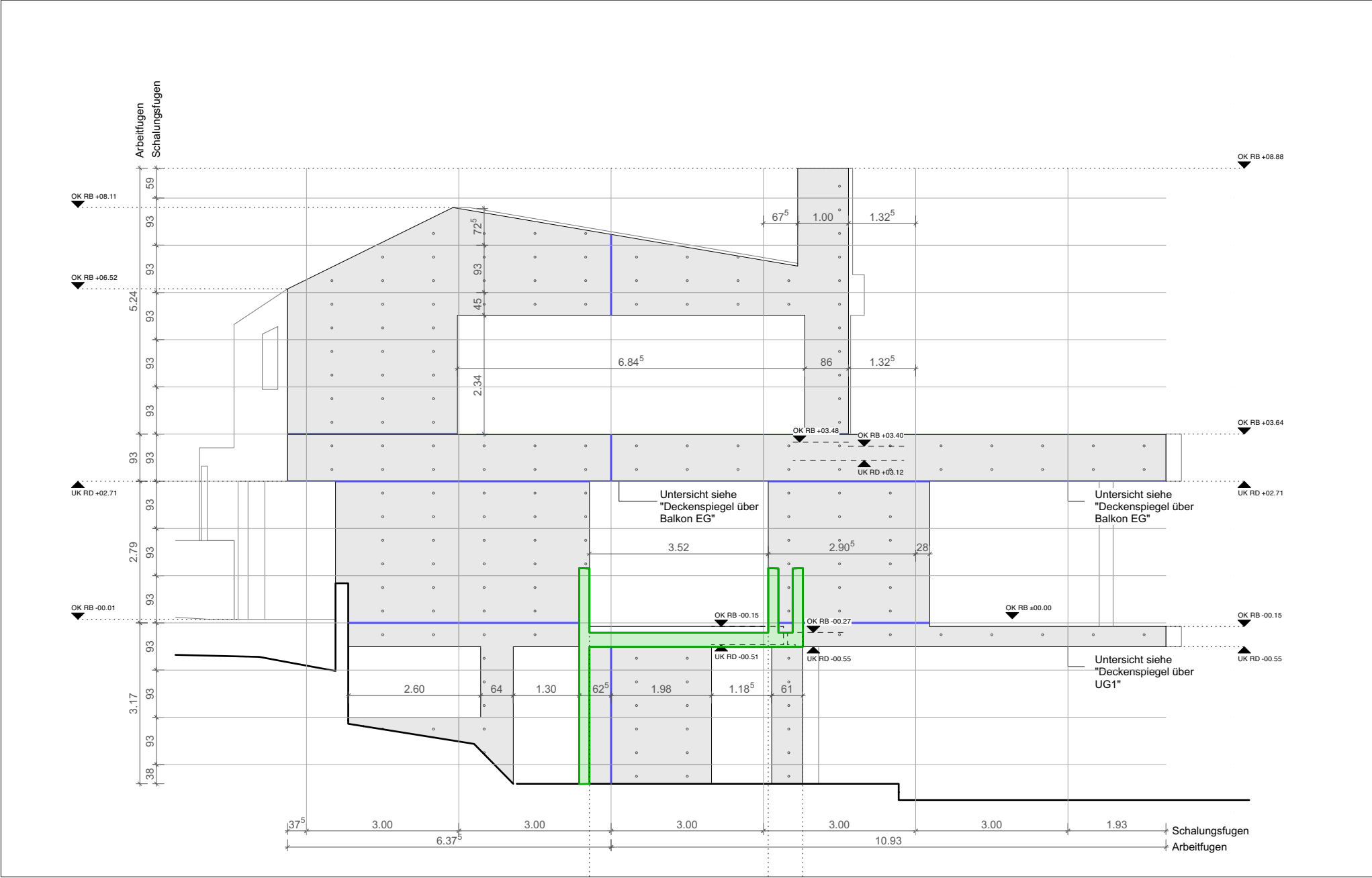
Hauptgebäude Ansicht West
