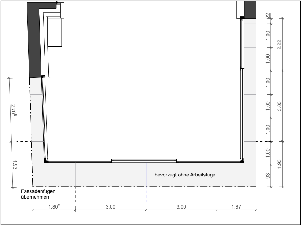
Deckenspiegel über Balkon EG
