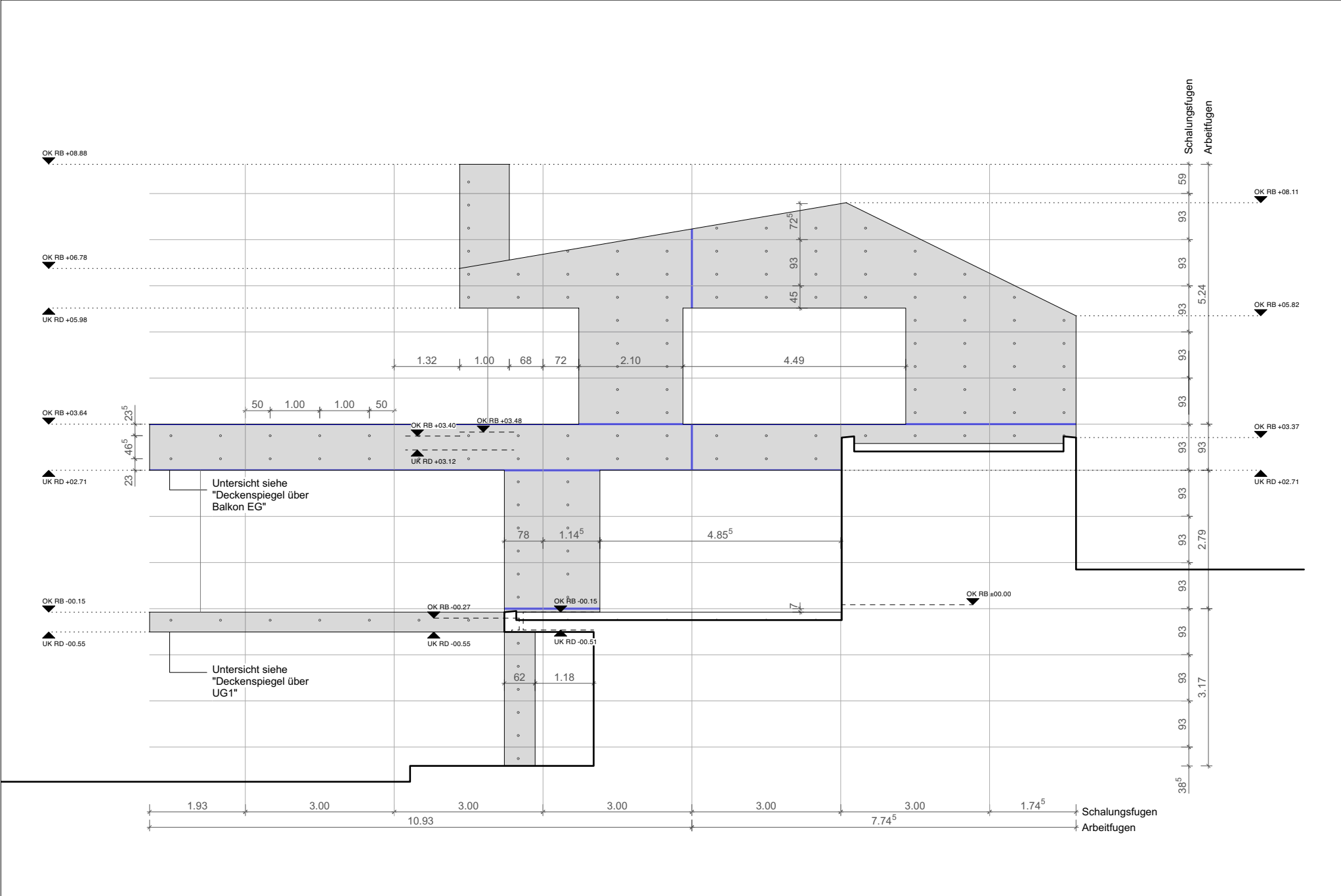
Hauptgebäude Ansicht Ost
