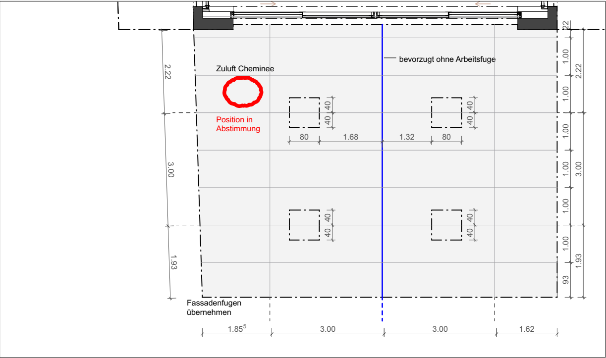
Deckenspiegel über UG1
