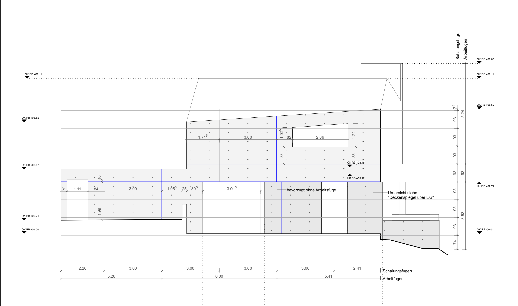
Hauptgebäude Ansicht Nord
