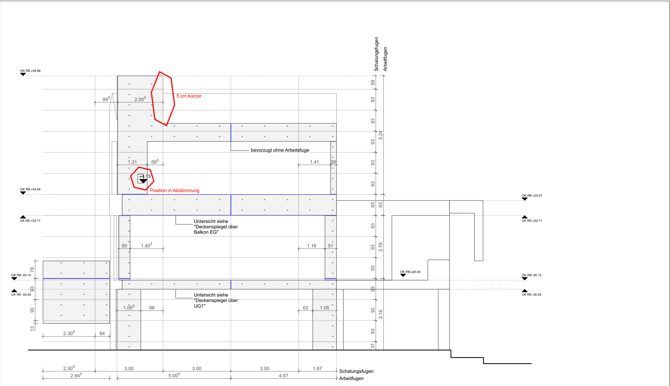
Hauptgebäude Ansicht Süd
