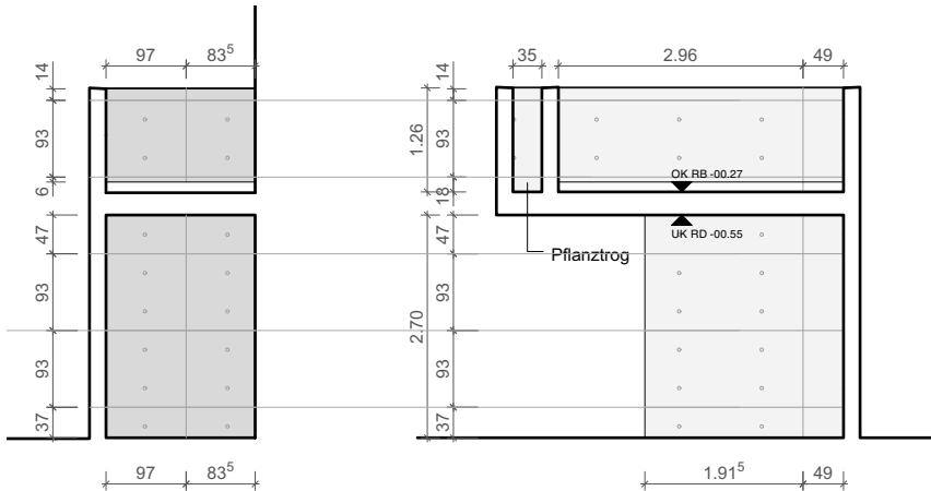
Ansicht Süd
