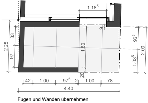
Deckenspiegel über UG1
