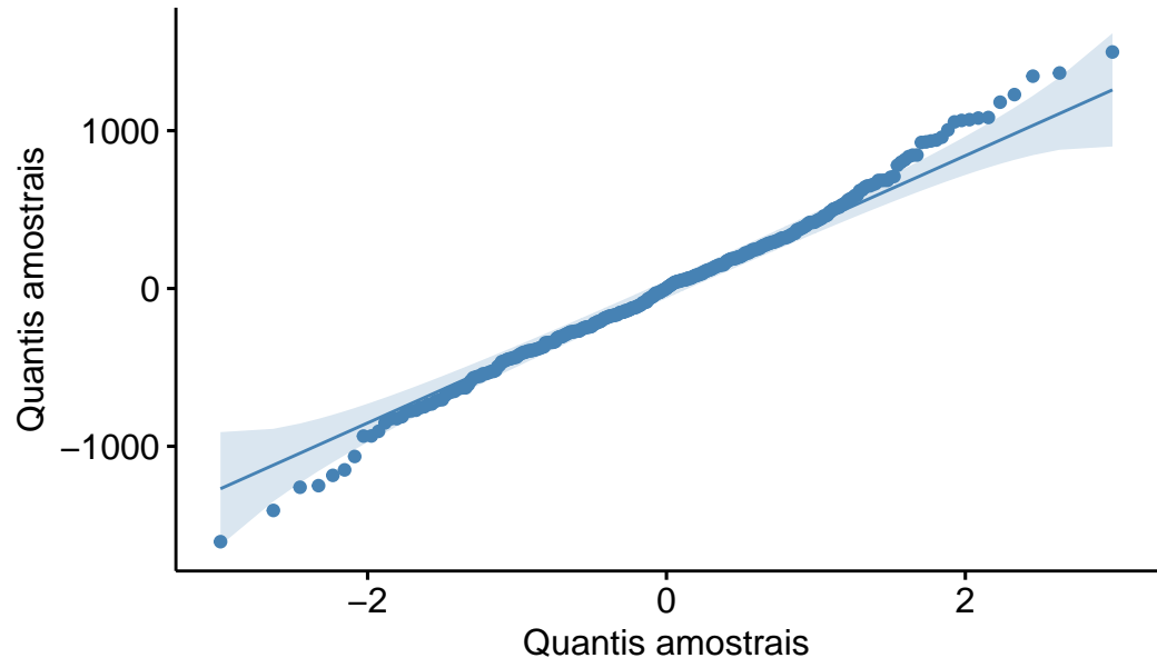
QQ Plot dos Resíduos
