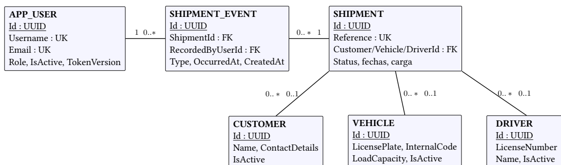
Figura 5.2: Modelo de datos implementado
