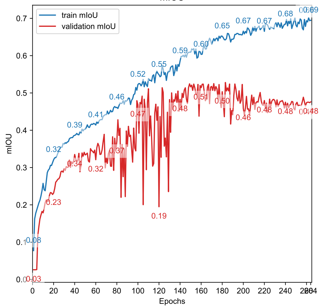
mIoU
