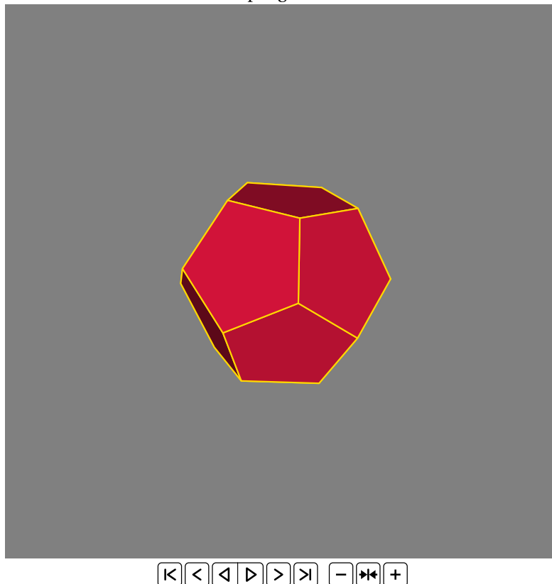
FIGURE 12 : Dépliage d'un dodécaèdre
