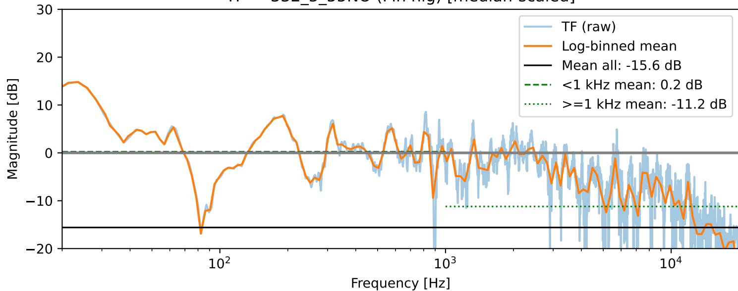
TF — 332_5_55NO (Pin nig) [median-scaled]
