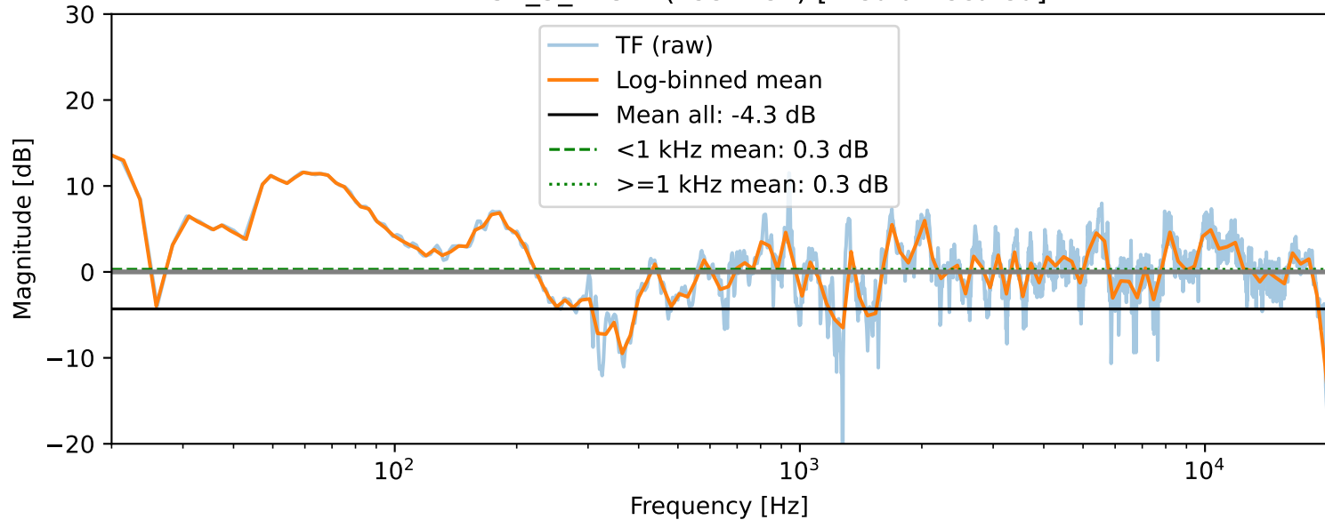
TF — 257_5_273W (Pse men) [median-scaled]
