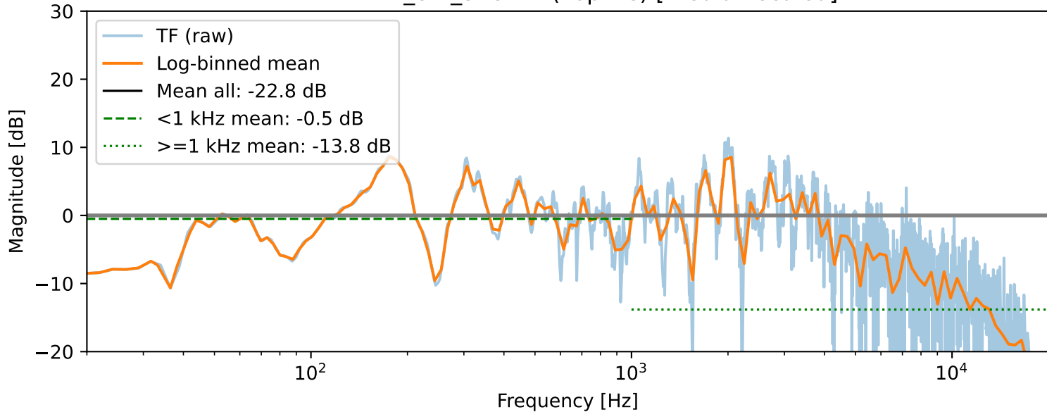
TF — 247_8.2_318NW (Pop tre) [median-scaled]
