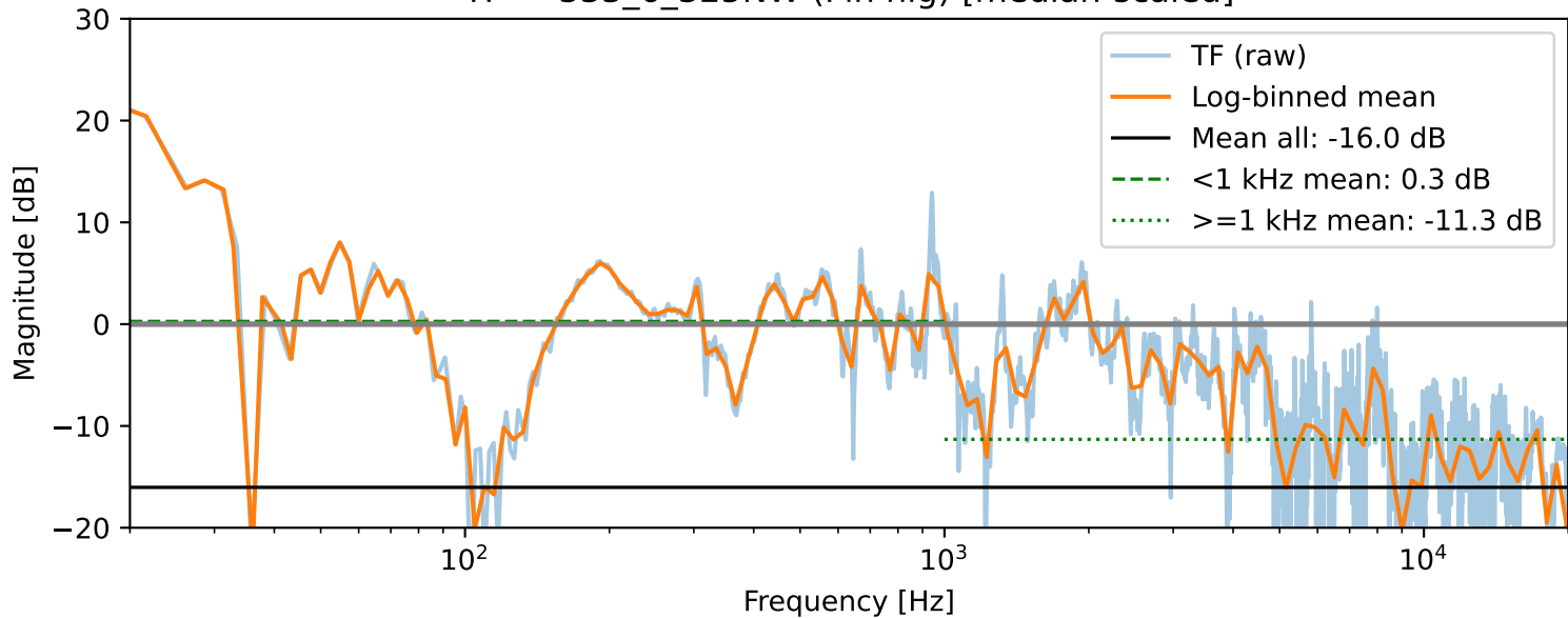
TF — 333_6_325NW (Pin nig) [median-scaled]
