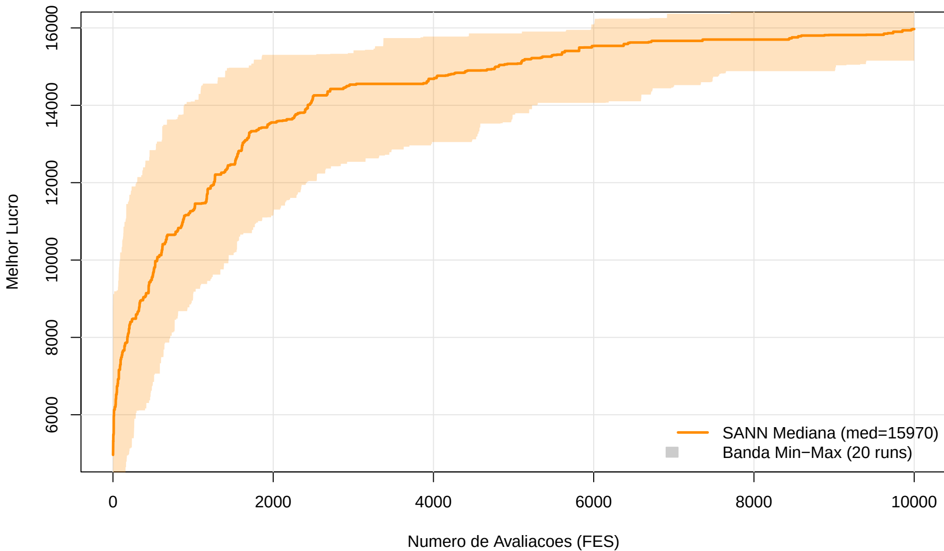
Convergencia SANN O1 (Mediana e Banda Min-Max) – T=500
