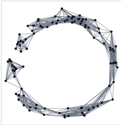
iKNN
