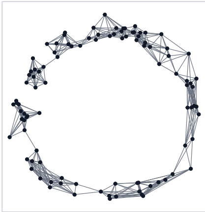
sKNN
