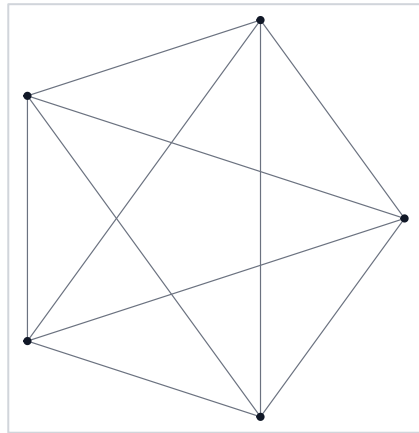
iKNN
