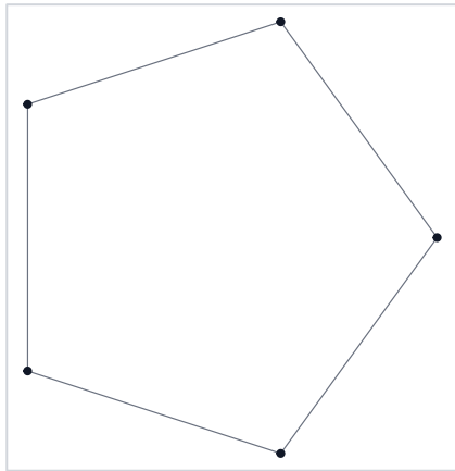
sKNN
