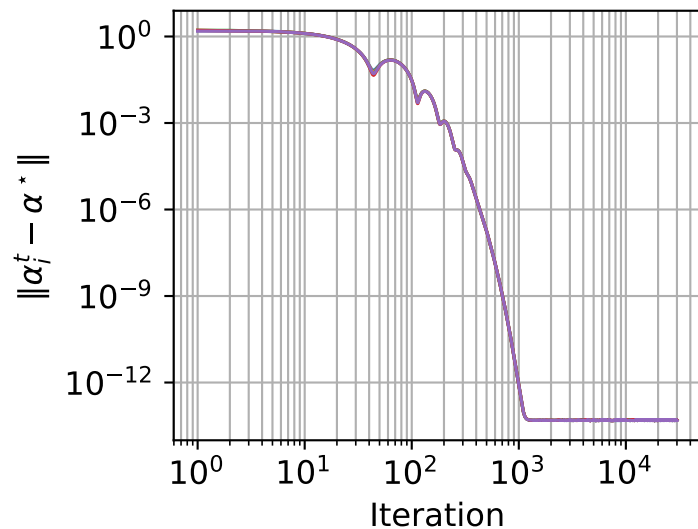
ADMM
