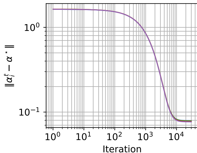
DGD
