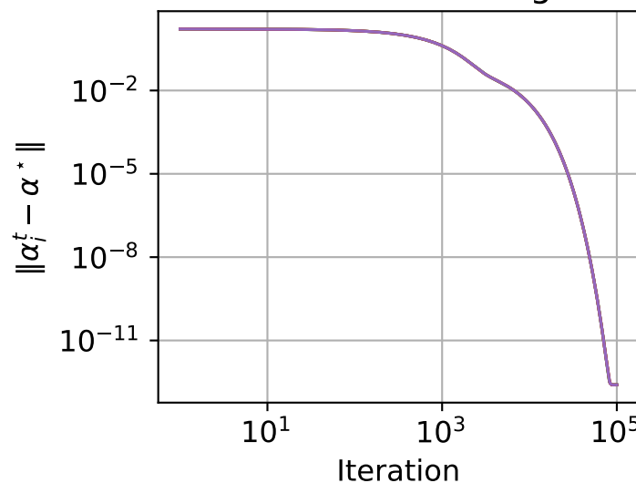
Gradient tracking
