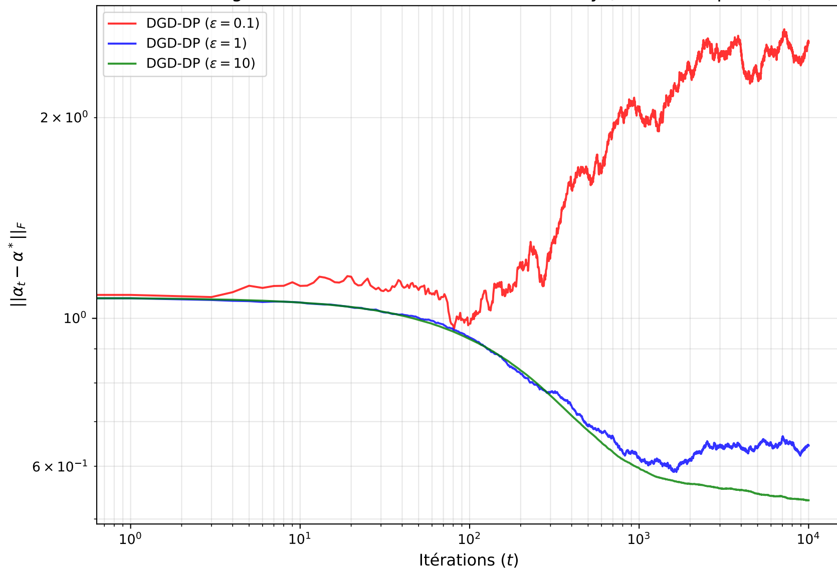
Convergence du DGD avec Differential Privacy (Bruit de Laplace)
