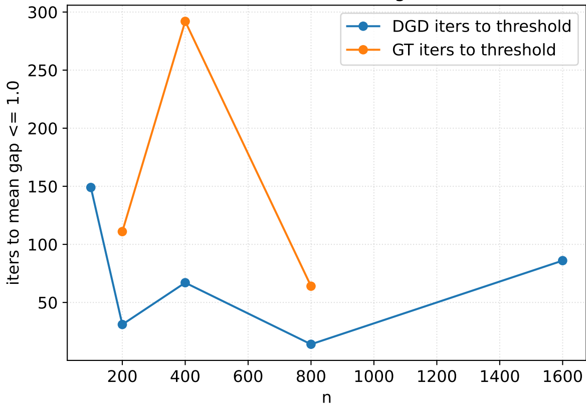
Part I - vitesse de convergence vs n
