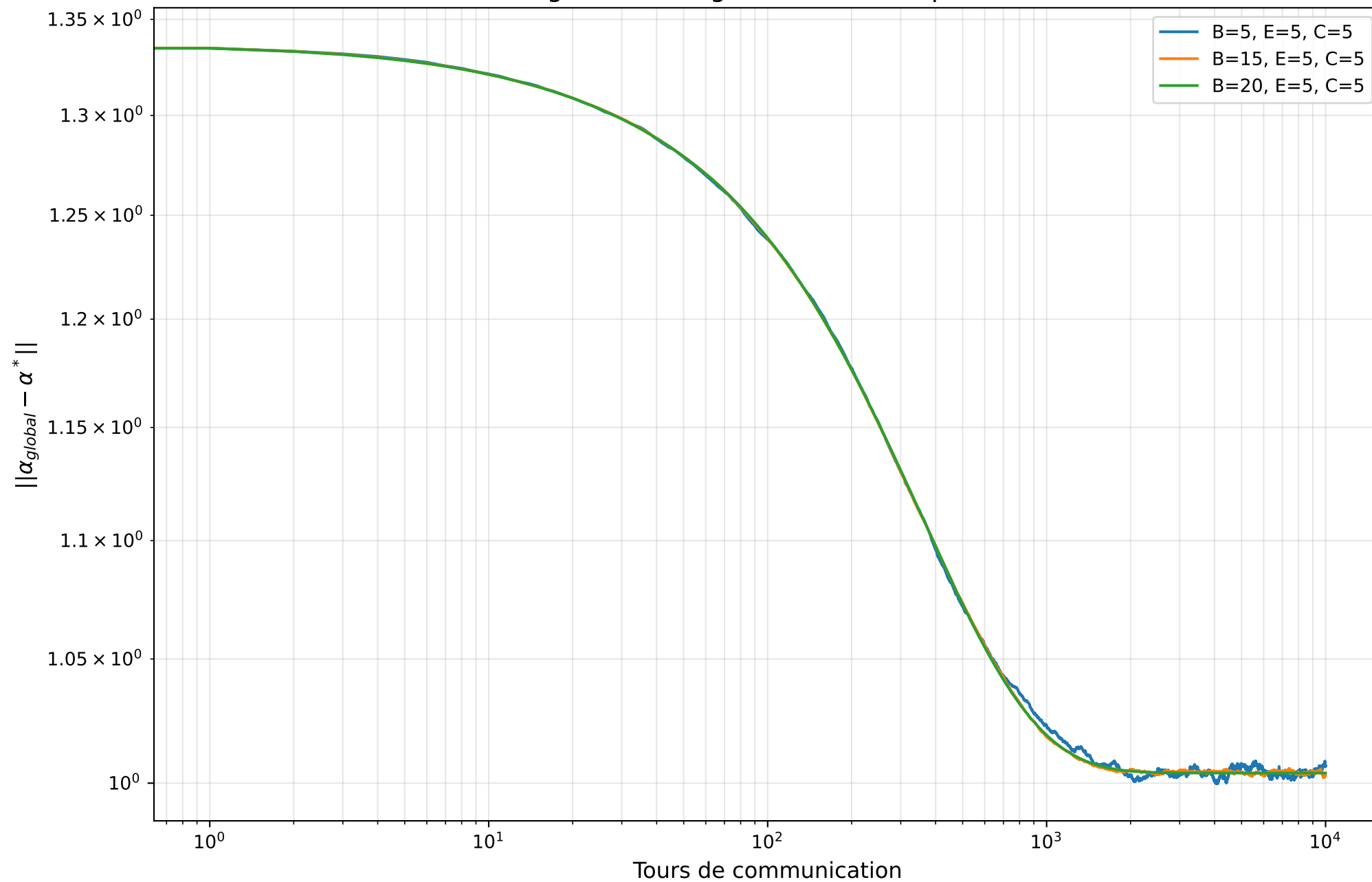
Convergence FedAvg : Influence des paramètres
