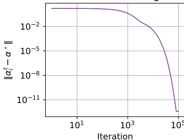
Gradient tracking
