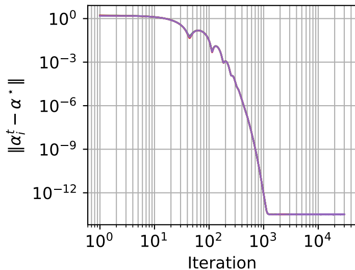
ADMM
