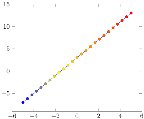
Default arguments
