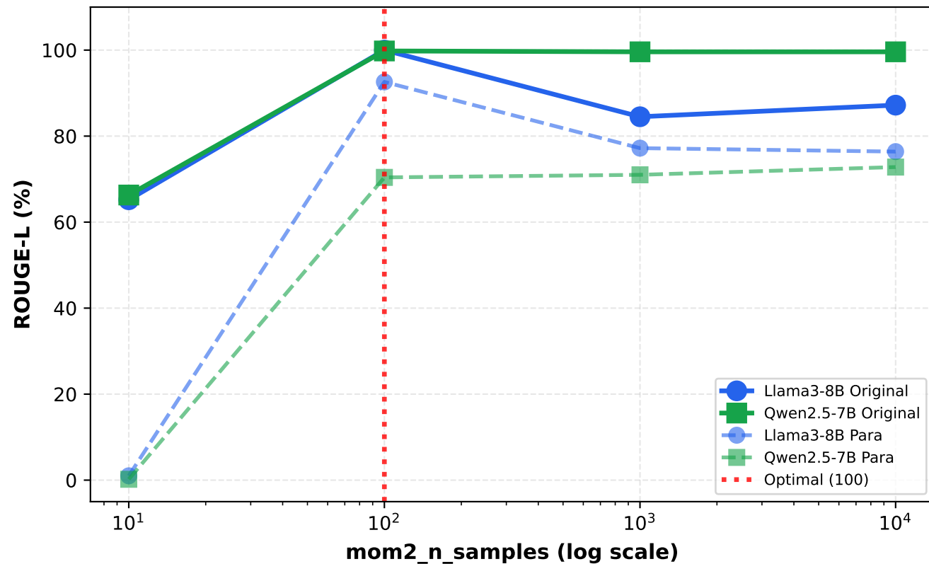
ROUGE-L Trends
