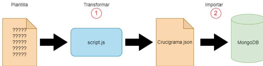
Figura 6: Transformación de la plantilla personalizada de la cuadrícula a una plantilla EJSON que puede leer MongoDB
