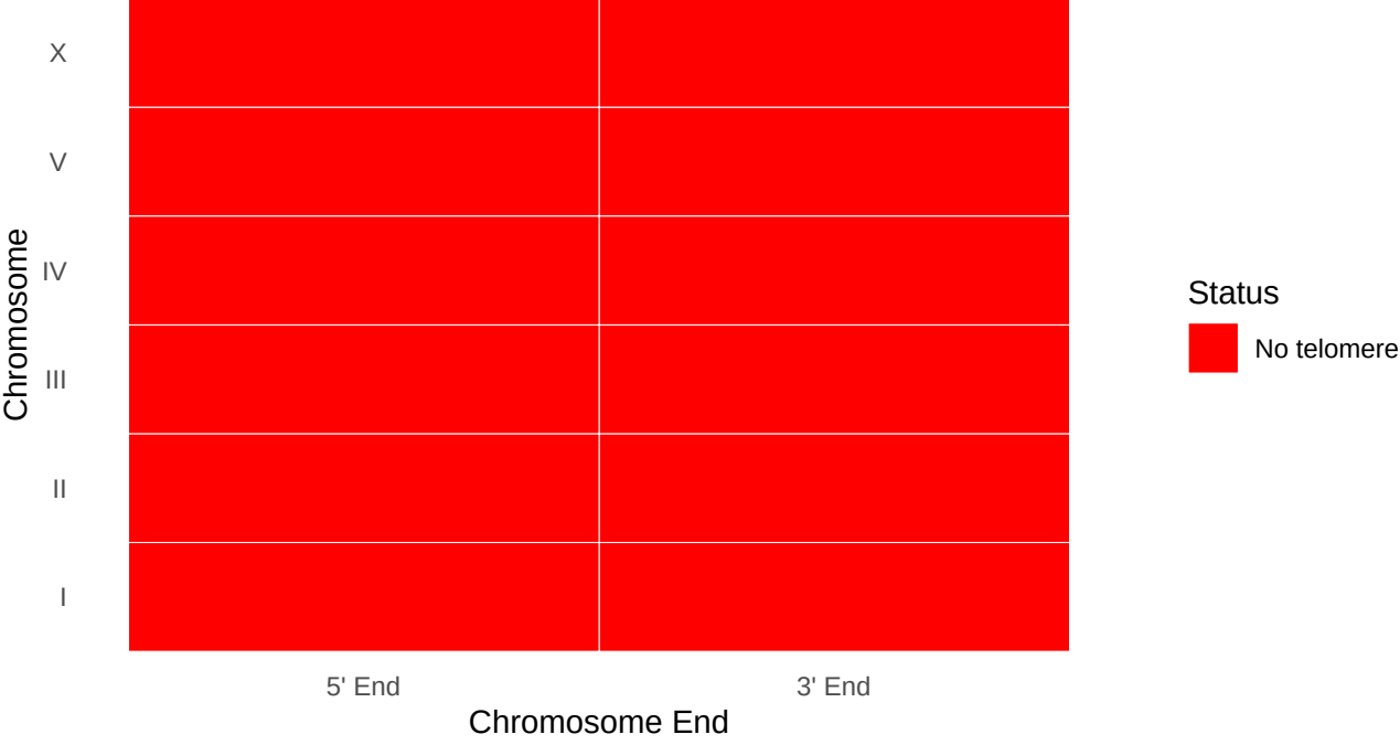
Telomere Status for Oscheius tipulae
