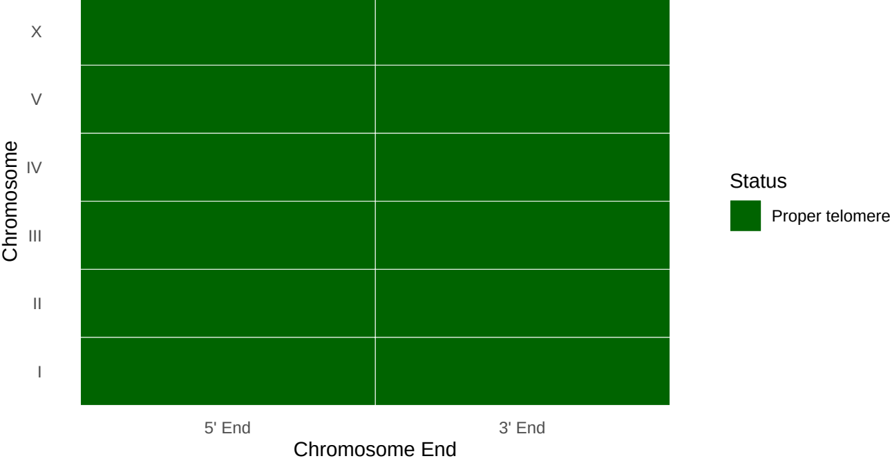
Telomere Status for Oscheius tipulae
