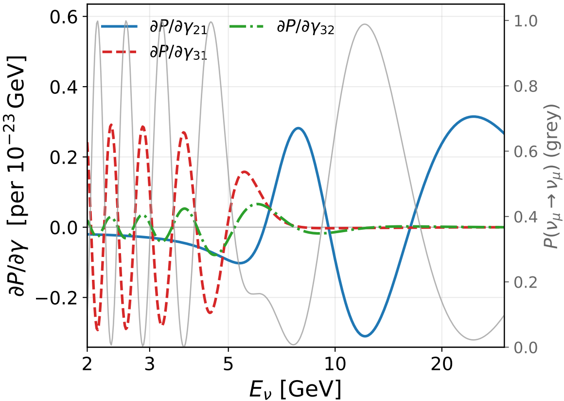
decoherence (Lindblad)
