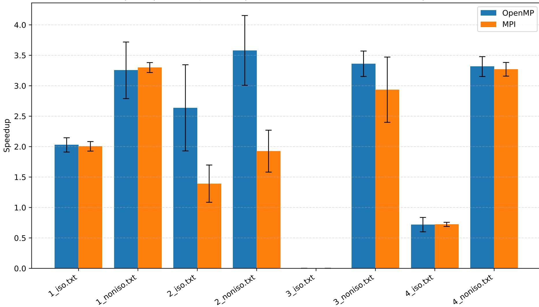
Speedup em relação ao sequencial com barras de erro de desvio padrão
