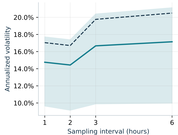
SPY
