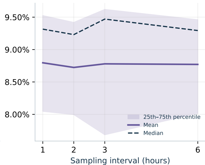
EUR/USD
