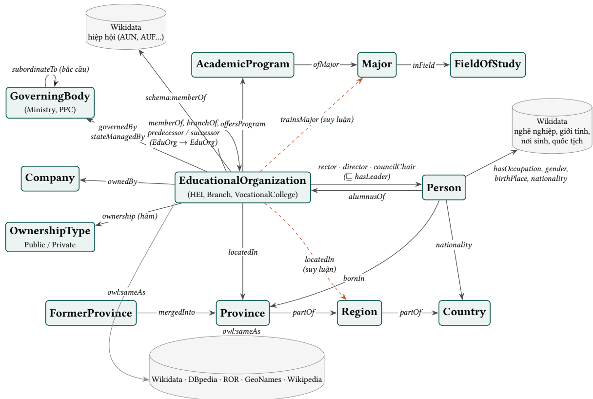
Hình 3. Đồ thị quan hệ của ontology vnedu: 2.1: nút là lớp, cạnh là quan hệ (miền → đích). Nét đứt: quan hệ suy luận; hình trụ: URI bên ngoài được tái sử dụng.
