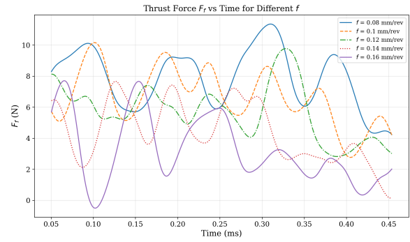
图 8: 图 3.8 不同进给量下进给抗力 (RF2) 随时间变化曲线
