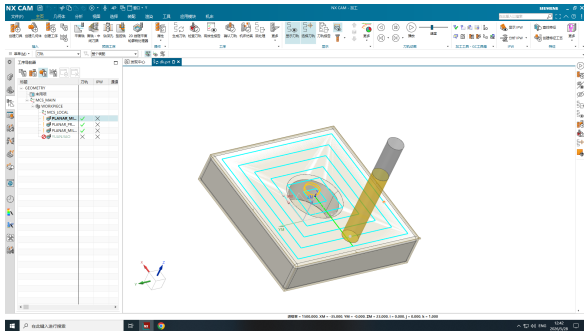
图 11: 图 4.3 NX CAM 刀具轨迹仿真
