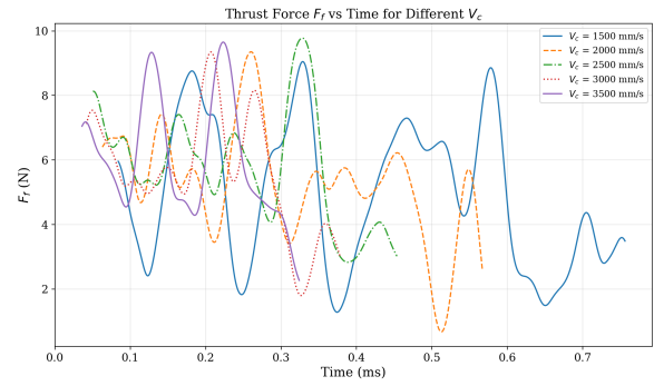
图 5: 图 3.5 不同切削速度下进给抗力 (RF2) 随时间变化曲线
