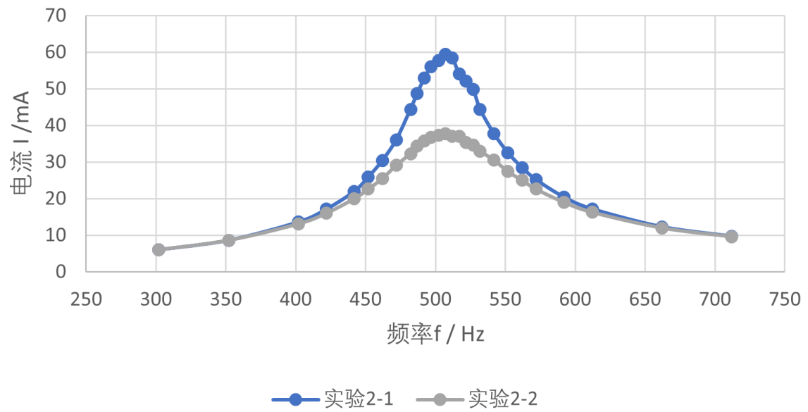
RLC 串联电路 I-f 曲线
