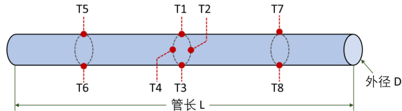
图 2 实验管热电偶布置图
