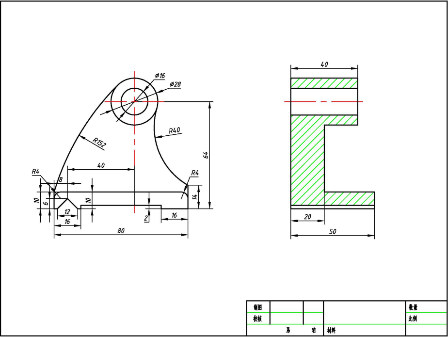
图 1 实验练习四的工程图
