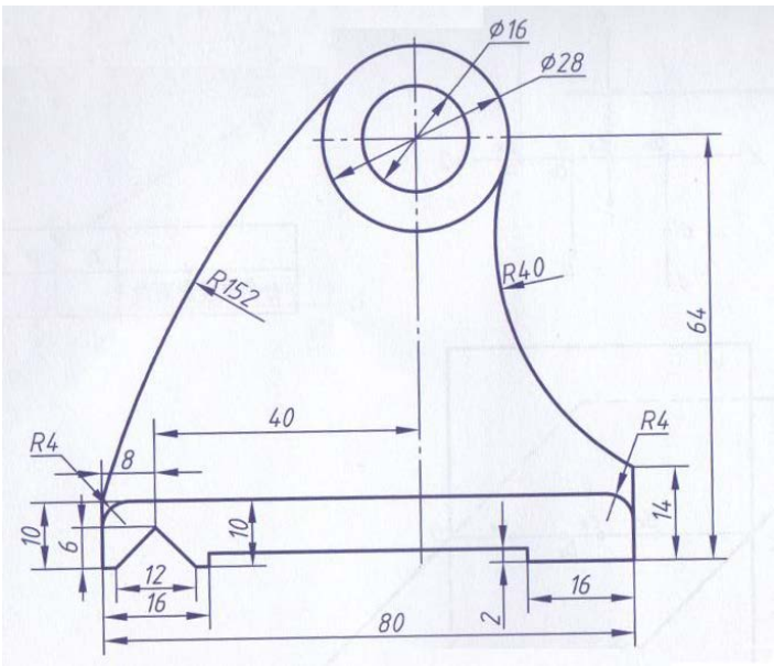
图 2 机械制图习题集 P3 练习 1-3-2
