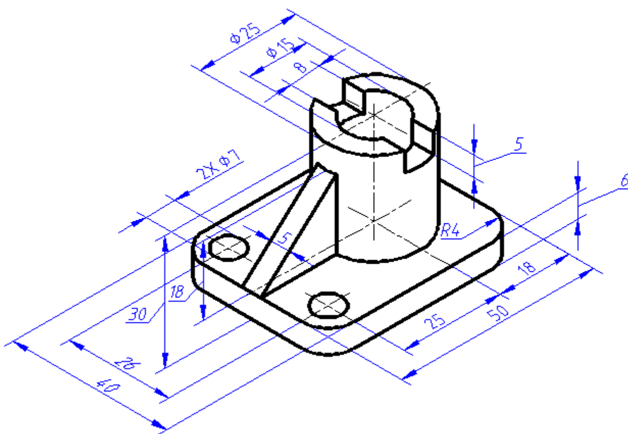
4-2-2-8 标注轴测图的尺寸（数值从图上按1:1量取）
