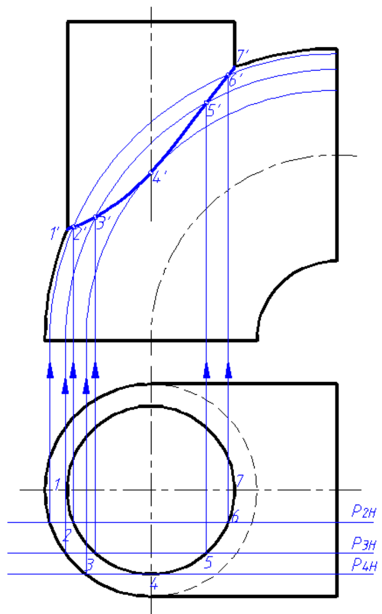
3-3-2-11 补全圆柱与圆环相交后视图中所缺的线。
