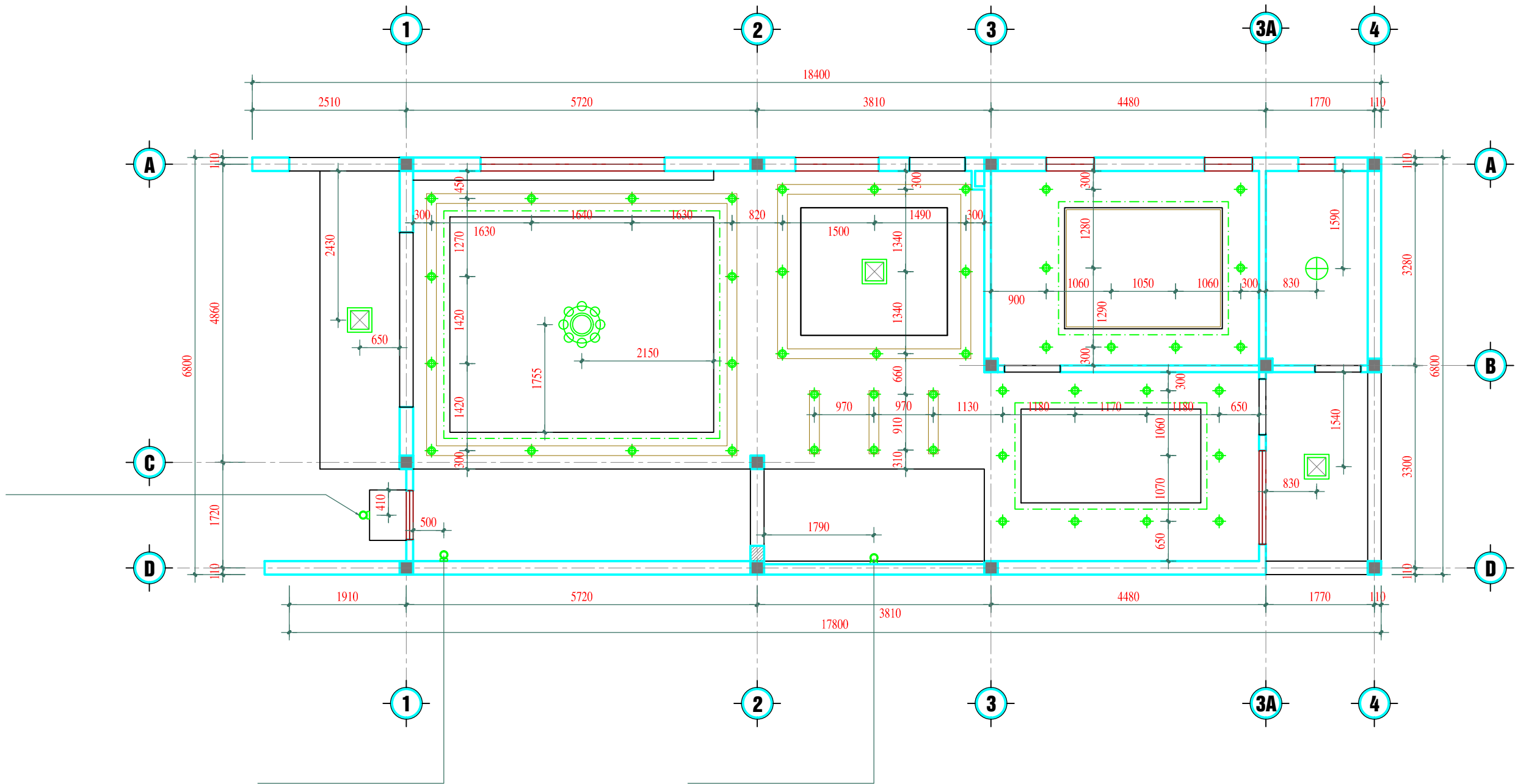
MẶT BẰNG ĐÈN TẦNG 1
