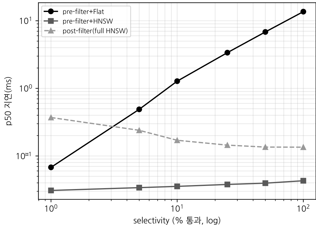
지연: pre-filter+Flat만 부분집합에 선형↑
