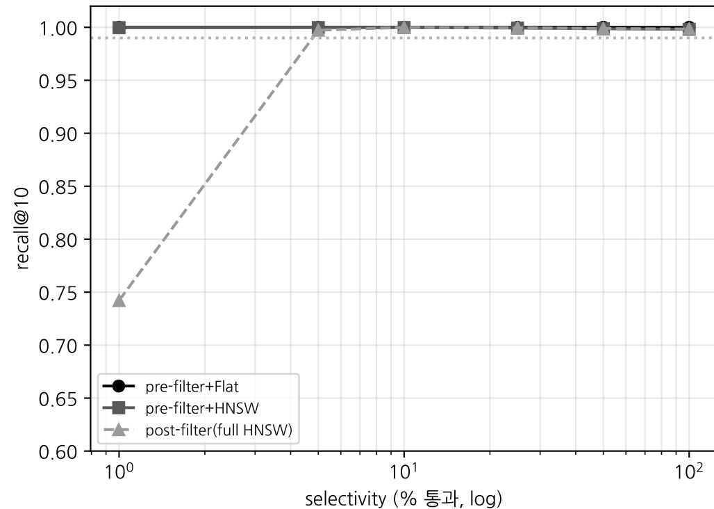
정확도: 고선택도에서 post-filter recall 붕괴
