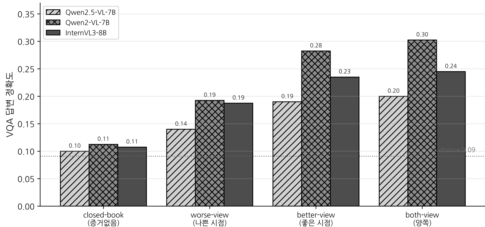
다각도 CCTV answer-level: 쌓기보다 선택 (n=400, 3개 VLM) better>worse 유의, both≈better(등가) — 서로 다른 vision encoder에서 반복
