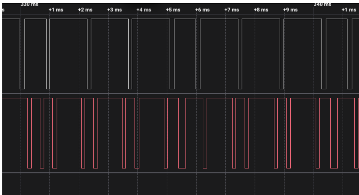
Figura 3: Inizio della prima trama della scheda in fig.1, separata in clock e dati
