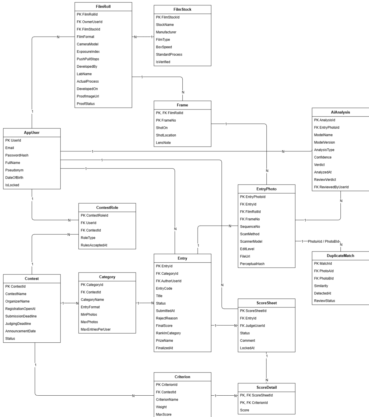
Hình 3.1: Sơ đồ thiết kế logic (Logical Diagram)
