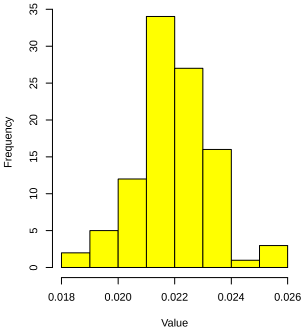
srmr
